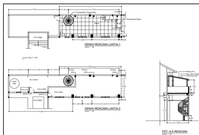
Gambar 2. Denah Rencana Pembangunan Gereja Katolik Salib Suci Tj. Anom
