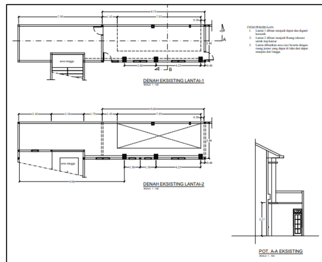
Gambar 1. Denah Existing Rumah Pastoral Tj. Selamat
